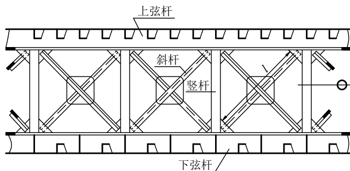
(1) 双向桁架
