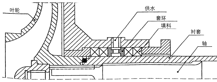
图 5.15.1.3 密封装置
