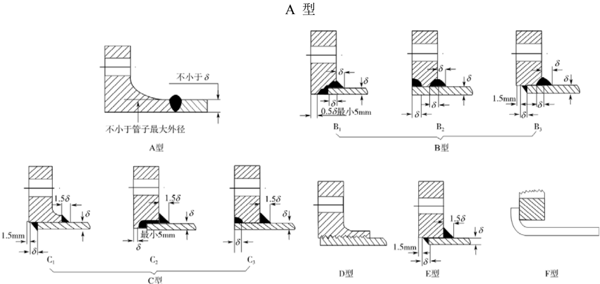
图 2.2.3.2 典型法兰连接
