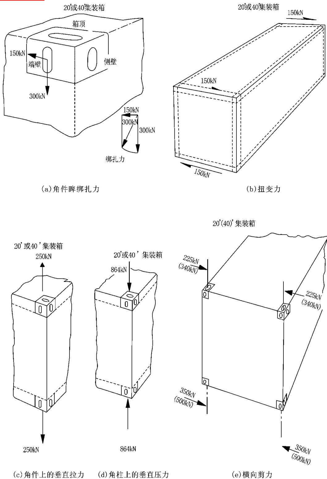
图 3.6.6.2 20'或 40'集装箱的许用负荷
